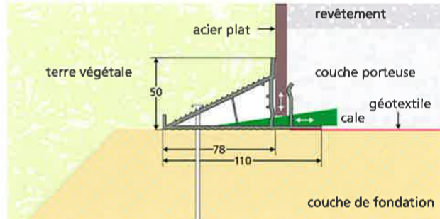
Section transversale de l'application.
